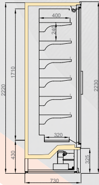
BONATITAN P/LB DGD 750/H2200
