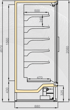
BONATITAN P/LB DGD 900/H2050
