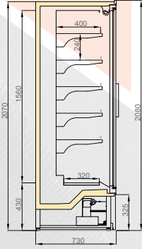
BONATITAN P/LB DGD 750/H2050
