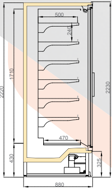
BONATITAN P/LB DGD 900/H2200
