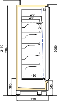
BONATITAN DGD 750/H2050
