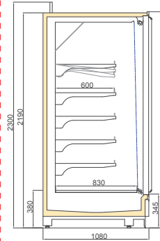
BONATITAN MT DGD 1100/H2200
