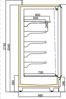
BONATITAN DGD 1000/H2050
