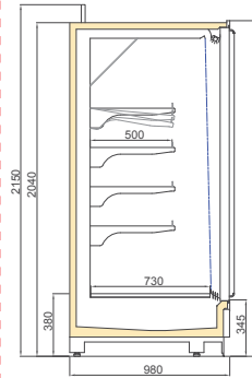
BONATITAN MT DGD 1000/H2050
