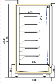
BONATITAN DGD 1100/H2200
