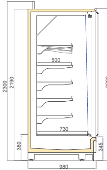
BONATITAN MT DGD 1000/H2200
