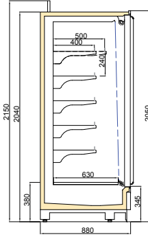
BONATITAN DGD 900/H2050
