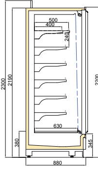
BONATITAN DGD 900/H2200
