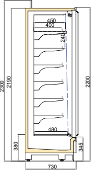
BONATITAN DGD 750/H2200
