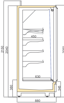
BONATITAN MT DGD 900/H2050
