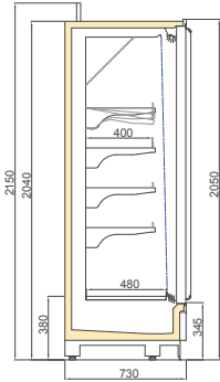
BONATITAN MT DGD 750/H2050
