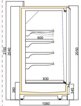
BONATITAN MT DGD 1100/H2050
