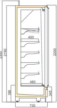
BONATITAN MT DGD 750/H2200
