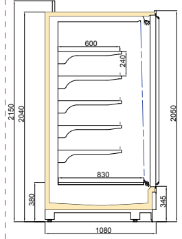
BONATITAN DGD 1100/H2050
