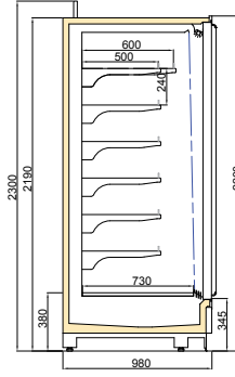
BONATITAN DGD 1000/H2200
